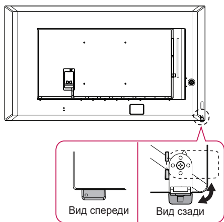
Монтаж в горизонтальном положении (по умолчанию)
