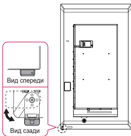
Монтаж в вертикальном положении
