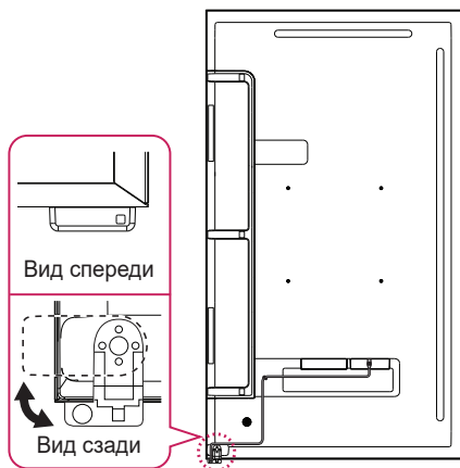
Монтаж в вертикальном положении
